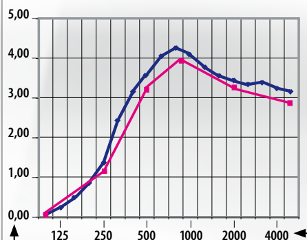
Schallabsorptionsgrad DIN EN 20354 Sound absorption ISO 354
